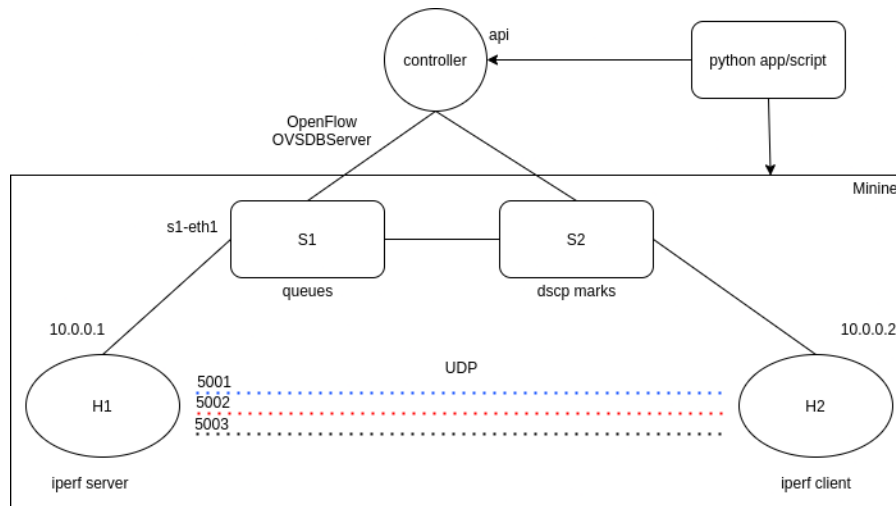
Figura 34: Esquema de laboratorio para ejecución de simulación de calidad de servicio. (Fuente: Elaboración propia)
