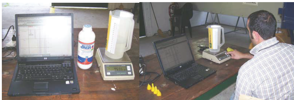
Figura 2.4. Determinaciones gravimétricas del volumen recolectado en el banco de distribución.
