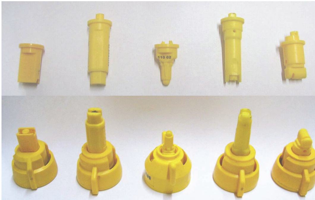
Figura 2.2. Pastillas de baja deriva asistidas por aire empleadas en la prueba. De izquierda a derecha: Agrotop Airmix Nodrift, Teejet Air Induction, Hypro Guardian AI, Lechler ID, Turbo Teejet Induction.
